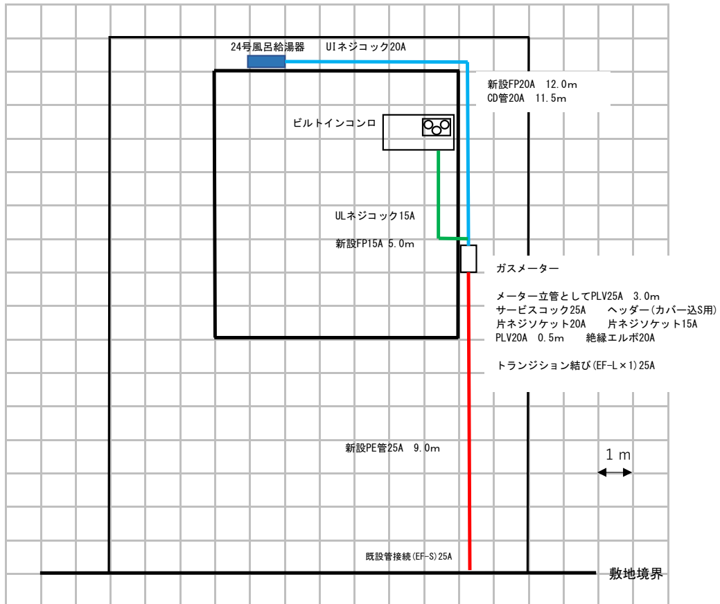
内管工事見積用平面図
