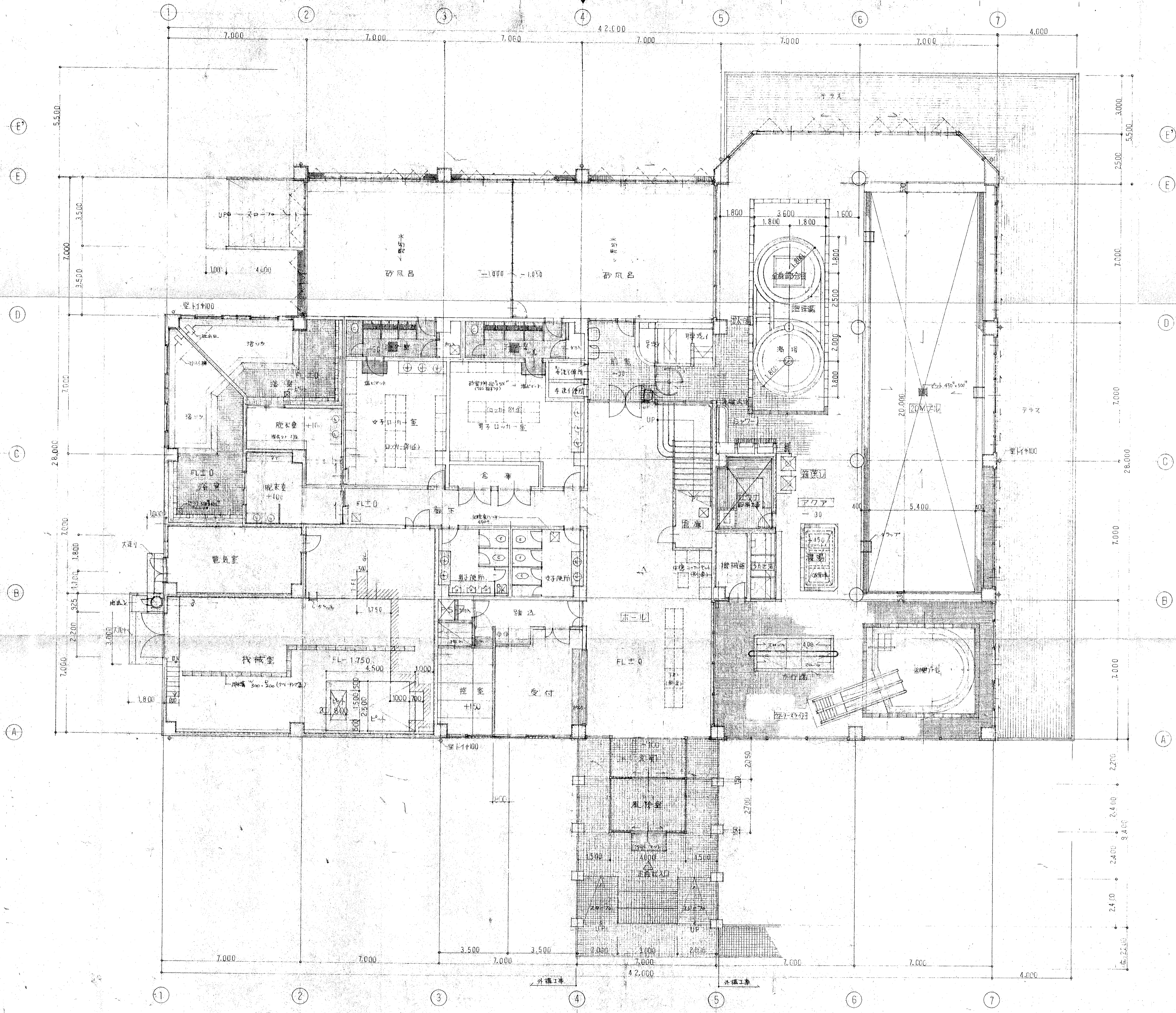
1階平面図 1/100
