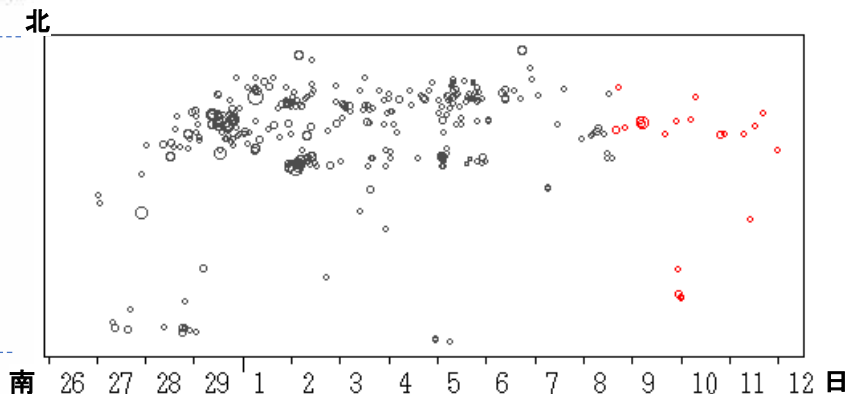
震央分布図の矩形内の時空間断面図
