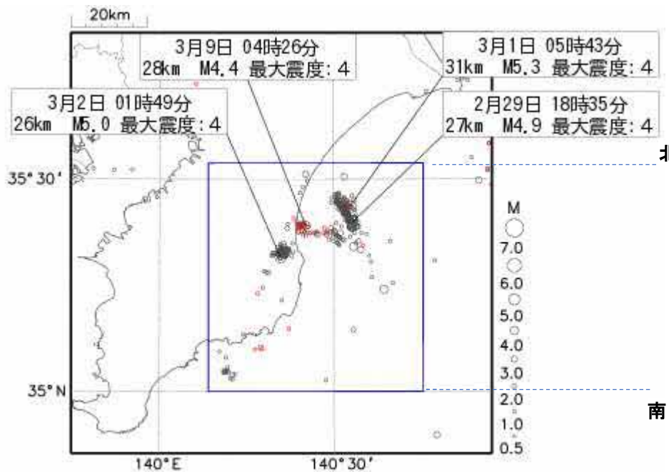
震央分布図
