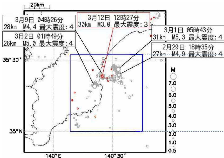
震央分布図
